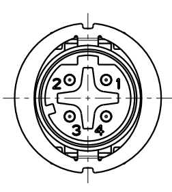
4pol D-Codierung (Steckseite) 4pole D-coding (Plug-in side)
