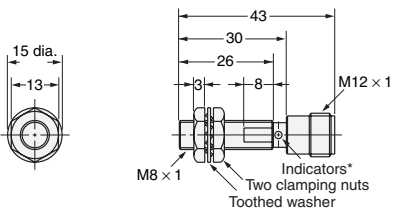
Diagram 18 E2E-X2D□-M1(G) E2E-X1R5E□-M1/E2E-X1R5F□-M1
