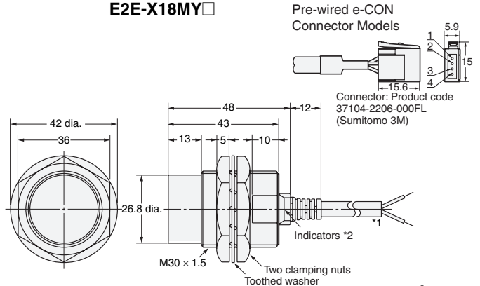
Diagram 17 E2E-X20MD□/E2E-X18ME□/F□ E2E-X18MY□
