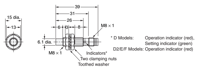
Diagram 29 E2E-X4MD□-M3G/E2E-X2ME□-M3/X2MF□-M3
