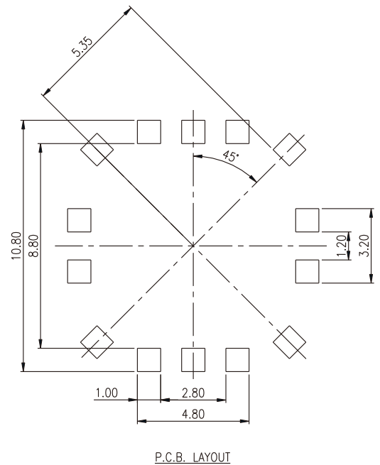
P.C.B. LAYOUT
