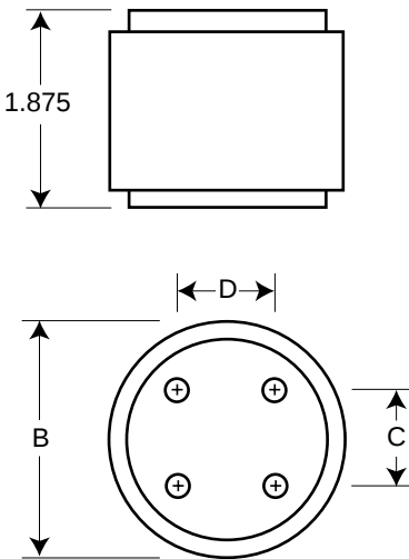
Fig. 2: 4000 Amp Range
