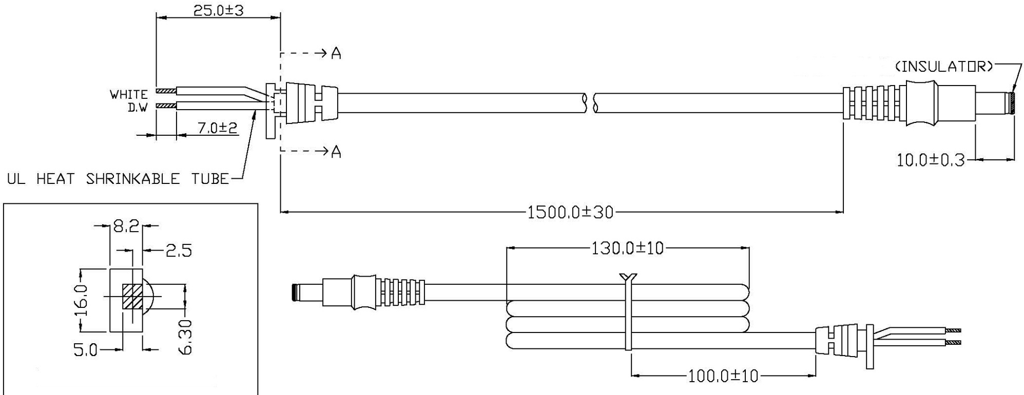
SECTION A-A
