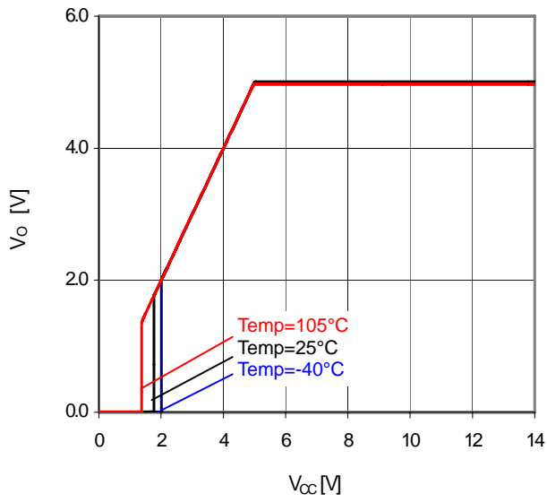
Fig.27 V_{CC}-V_o ( I_o=0\text{mA} )
