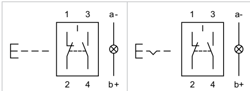
Wiring diagram 24
