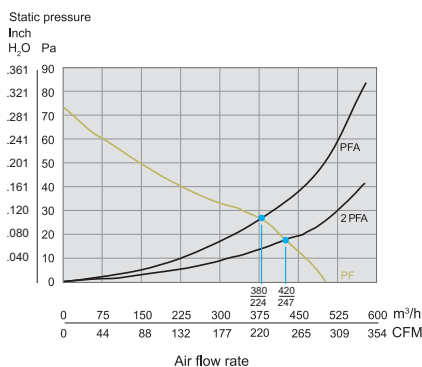
PF 65.000 IP55 / PFA 60.000 IP55
