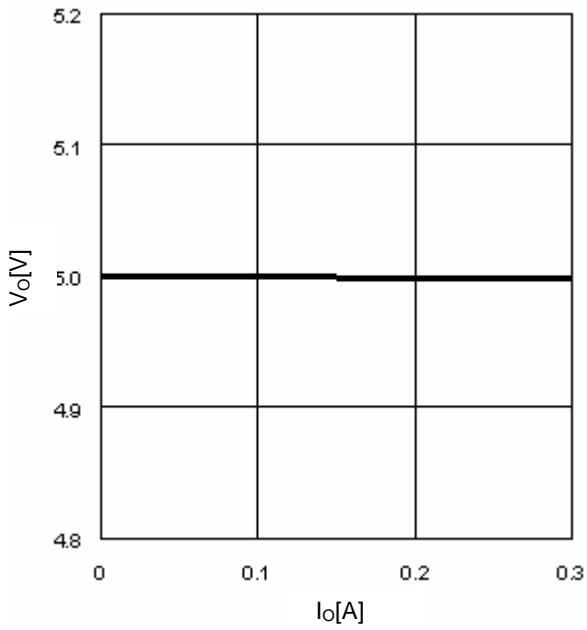
Figure 25. I O -V O
