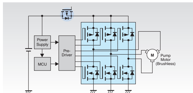
Brushless motor application ブラシレスモータタイプ
