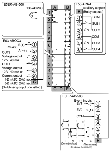
E5ER-Q43B-FLK
