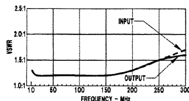
Input/Output VSWR
