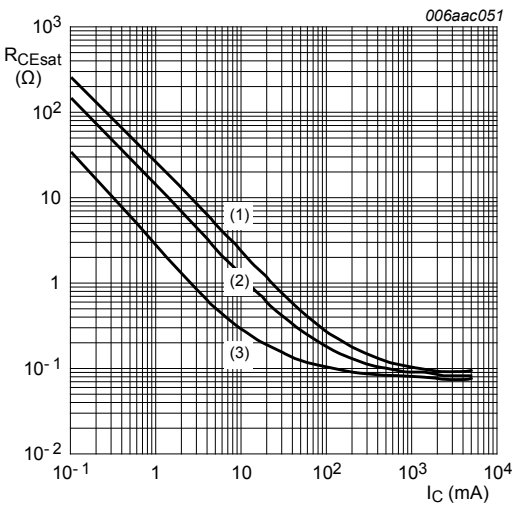
T_{amb} = 25\text{ °C} (1) I_C/I_B = 100 (2) I_C/I_B = 50 (3) I_C/I_B = 10
