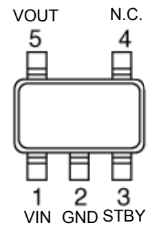
SSOP5(Top view)
