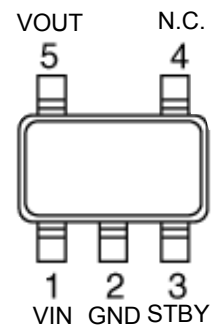
SSOP5(Top view)
