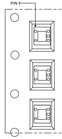
Fig. 13 - Taping Direction
