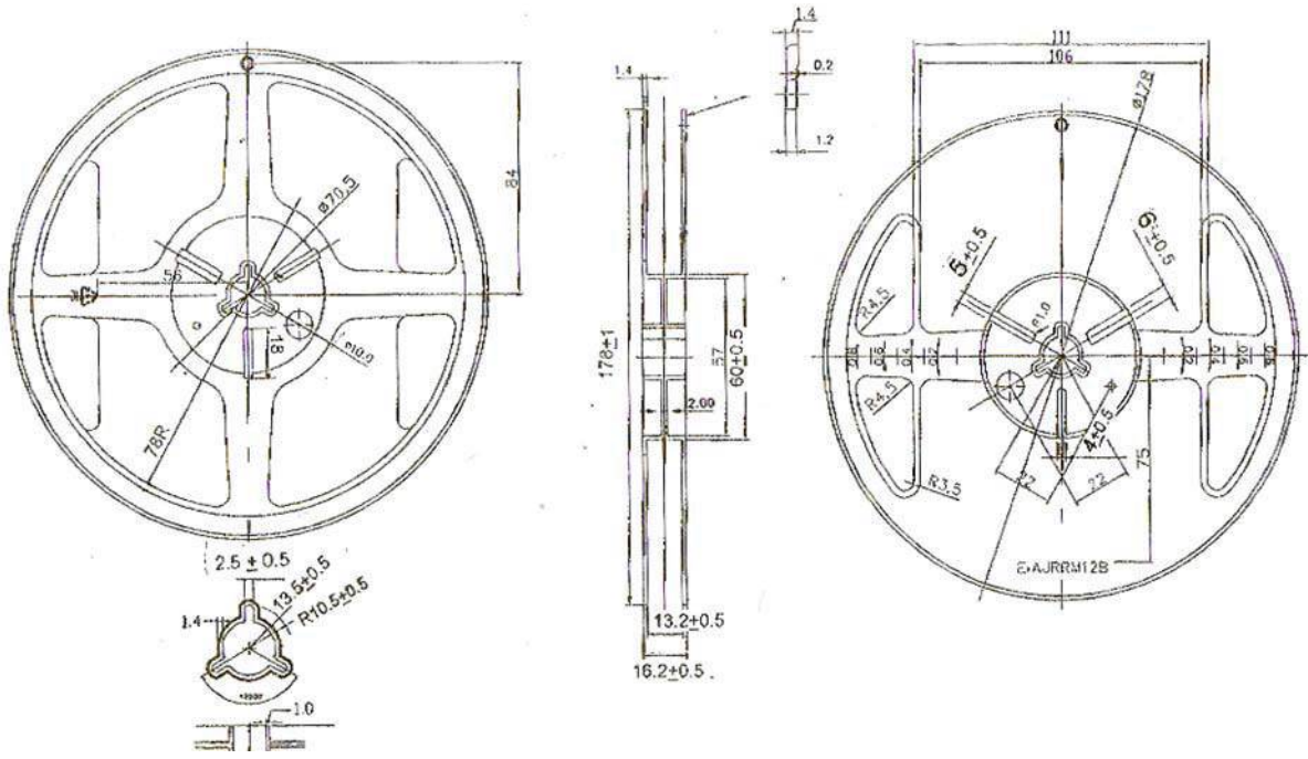
Fig. 14 - Reel Dimensions
