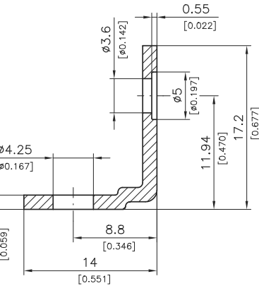
Metal Bracket F1080-23 Metallwinkel F1080-23
