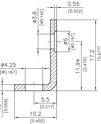
Metal Bracket F1080-18 Metallwinkel F1080-18
