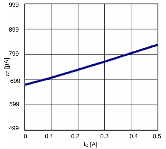
Fig.19 I_o - I_{cc}
