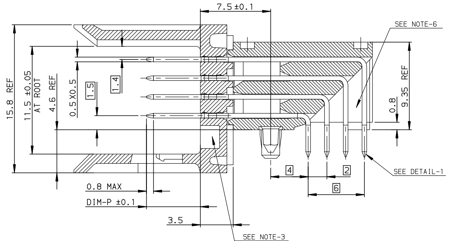
SECTION-A SCALE:4/1
