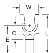
M18-10FL
