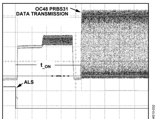
Figure 14. ALS Negate Time, 200\mu\text{s}/\text{DIV}
