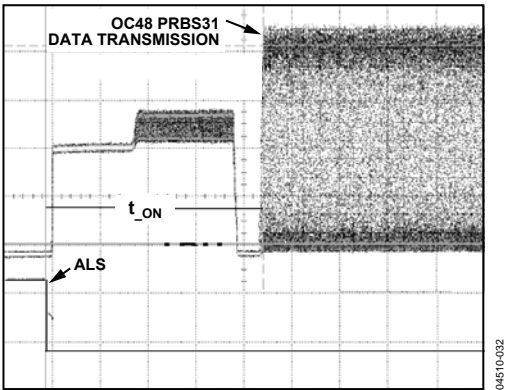
Figure 14. ALS Negate Time, 200\text{ }\mu\text{s/DIV}
