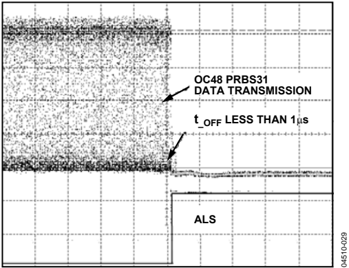
Figure 13. ALS Assert Time, 5\text{ }\mu\text{s/DIV}
