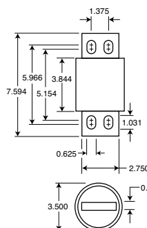
Fig. 2: 900-1000A
