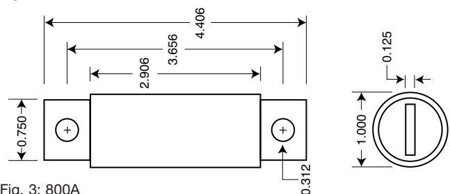
Fig. 3: 800A
