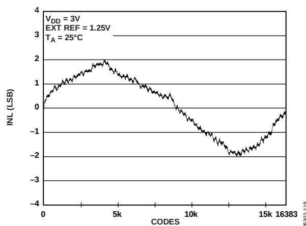
Figure 20. INL AD5648-1
