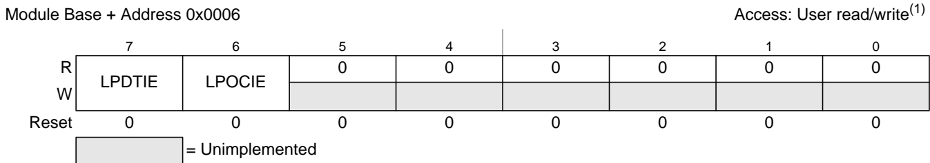
Figure 18-9. LIN Interrupt Enable Register (LPIE)
