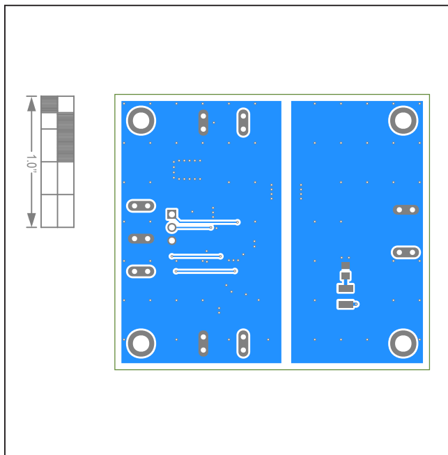
MAX17686EVKITA# - Bottom
