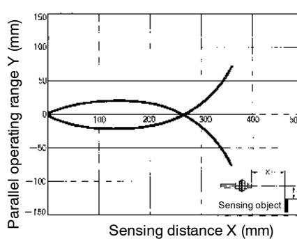
E32-D11L with E3X-H11 amplifier
