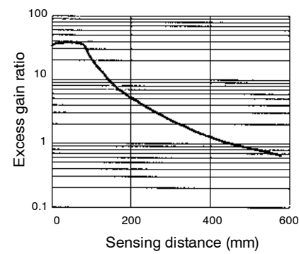
E32-T51 with E3JU-XR amplifier
