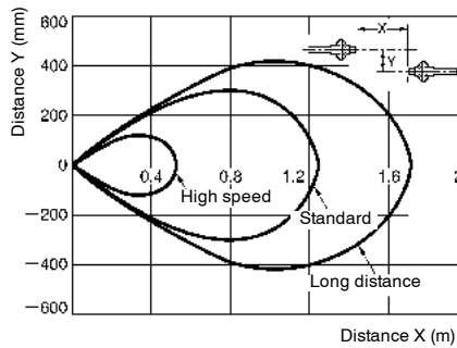
E32-T11 with E3X-NH amplifier
