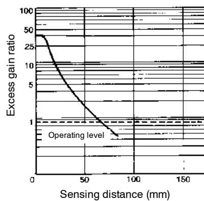
E32-TC200E with E3X-A11 amplifier
