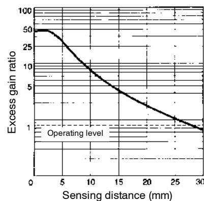
E32-TC200 with E3X-DA amplifier
