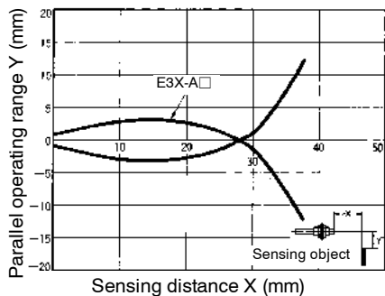
E32-DC200E with E3X-A11 amplifier
