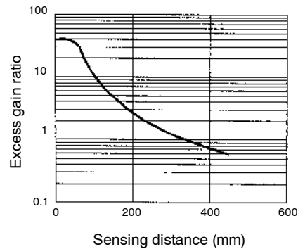
E32-TC200A with E3X-A11 amplifier
