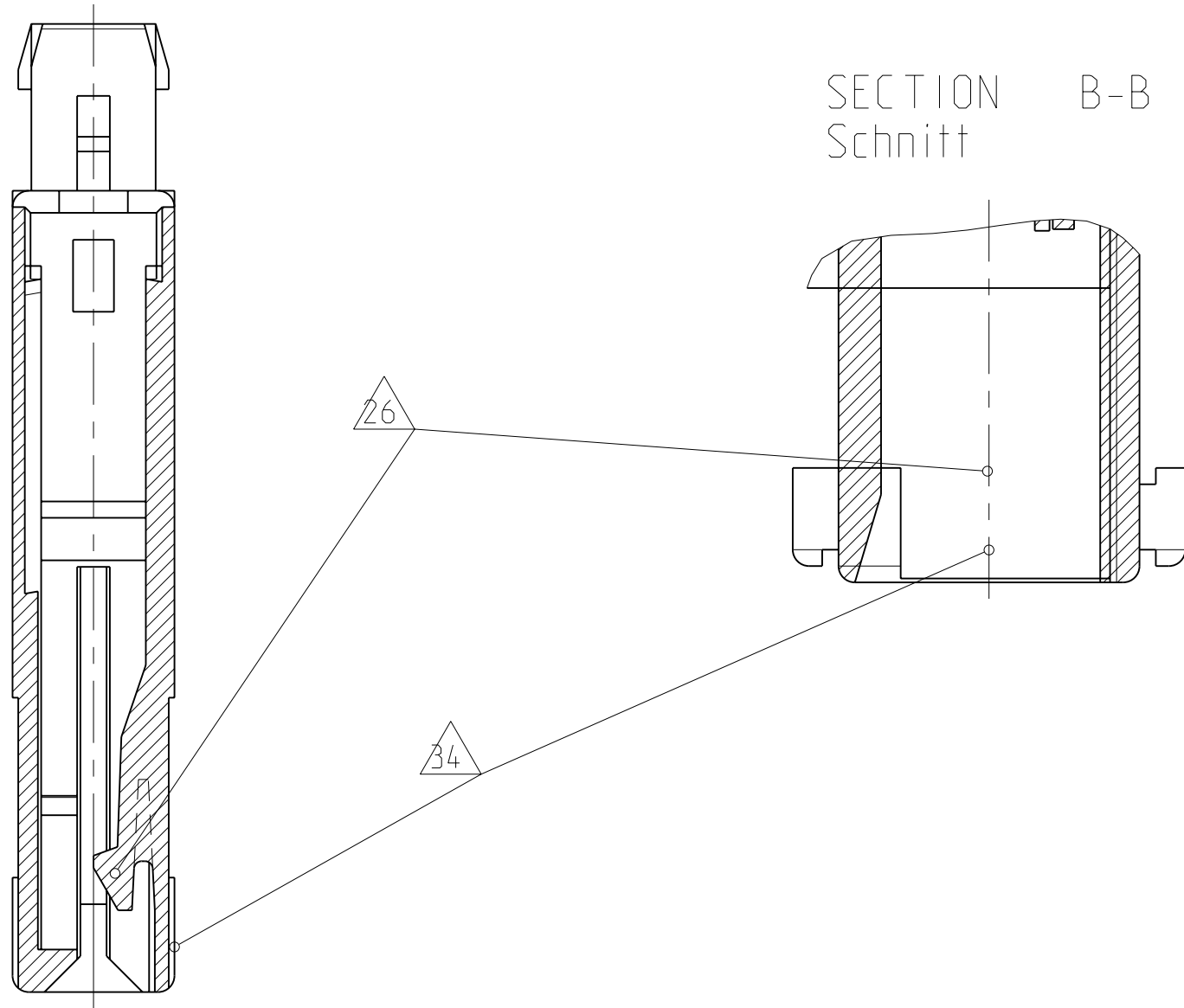
SECTION A-A Schnitt WITHOUT CONTACT Ohne Kontakt
