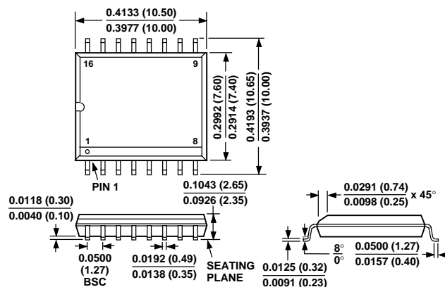
SOIC (R-16)
