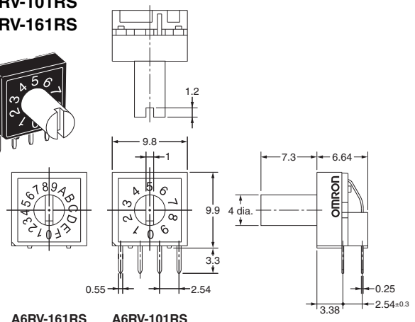
A6RV-161RS
