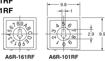
A6R-161RF
