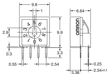
A6RV-101RF
