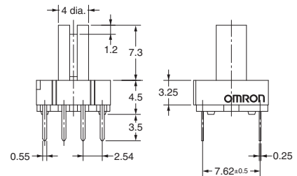
A6R-101RS
