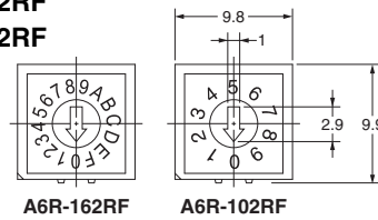
A6R-162RF
