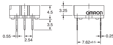
A6R-102RF
