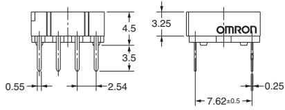
A6R-101RF
