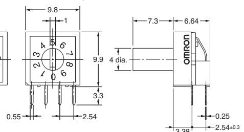
A6RV-101RS
