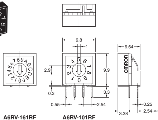
A6RV-161RF
