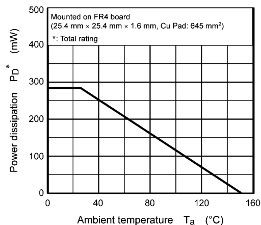
Fig. 7.14 P_D - T_a
