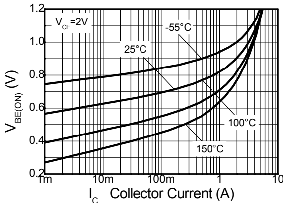
V_{BE(ON)} \text{ } v \text{ } I_C
