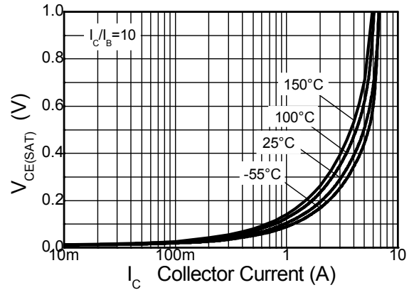
V_{CE(SAT)} \text{ } v \text{ } I_C
