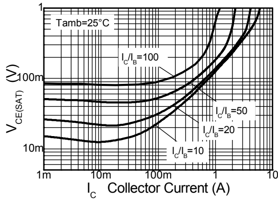
V_{CE(SAT)} \text{ } v \text{ } I_C
