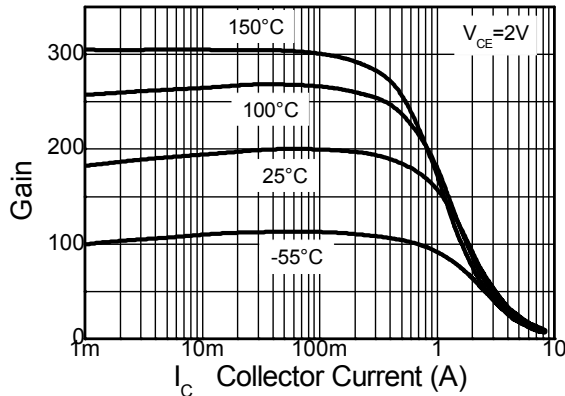
h_{FE} \text{ } v \text{ } I_C
