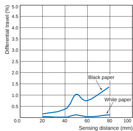
E3Z-LS□3/LS□8
