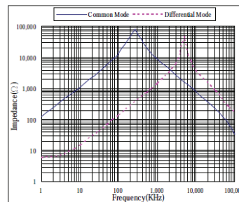
ALFT-09V-103
