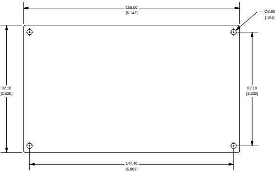
ENCLOSURE LID
