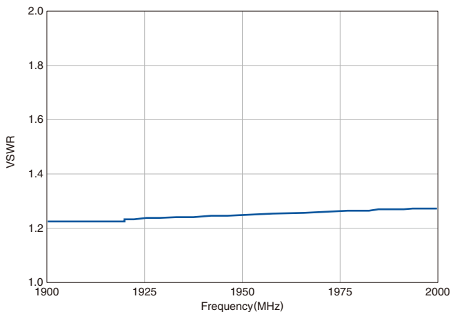
VSWR
