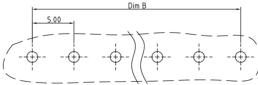
P.C.B. LAYOUT
