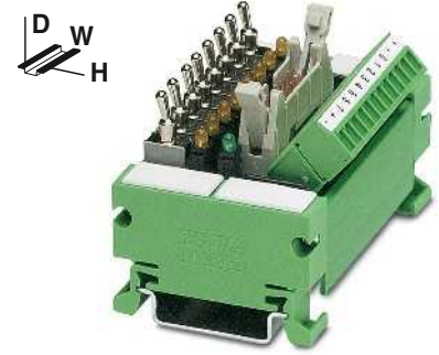
Switch module
