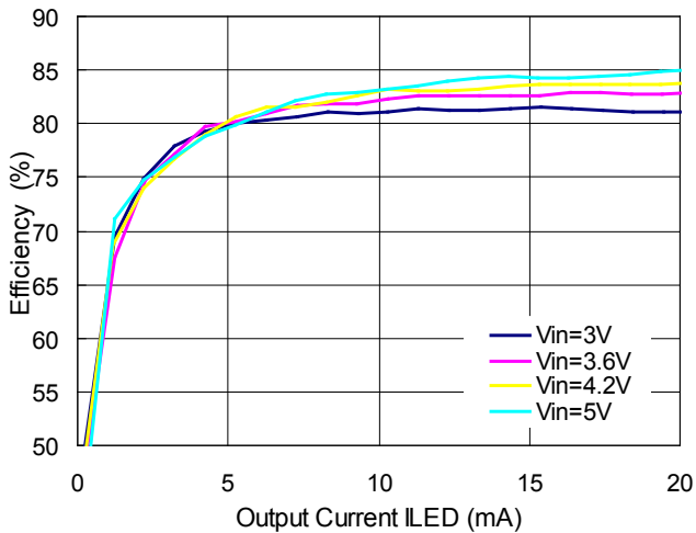
4LED, L=10\mu H (LQH32CN100K53)
