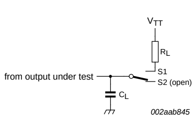
a. Load circuit
