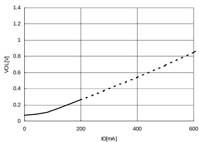
IO-VOL VDD=12V
