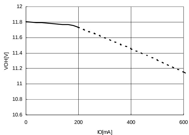
IO-VOH VDD=12V
