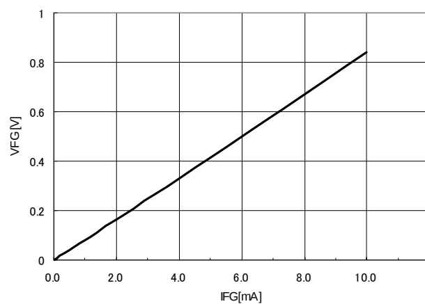
VFG-IFG VDD=12V
