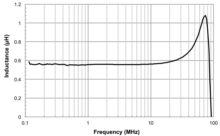
MPI4020V2-R56-R
