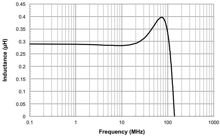
MPI4012V2-R33-R
