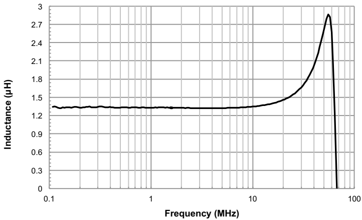
MPI4012V2-1R5-R
