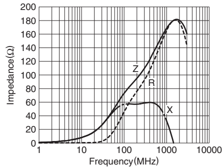
MMZ0603Y471C
