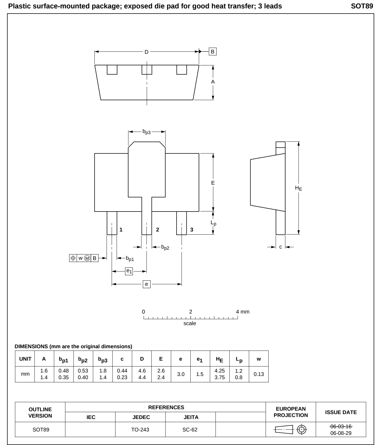
Fig 27. Package outline SOT89
