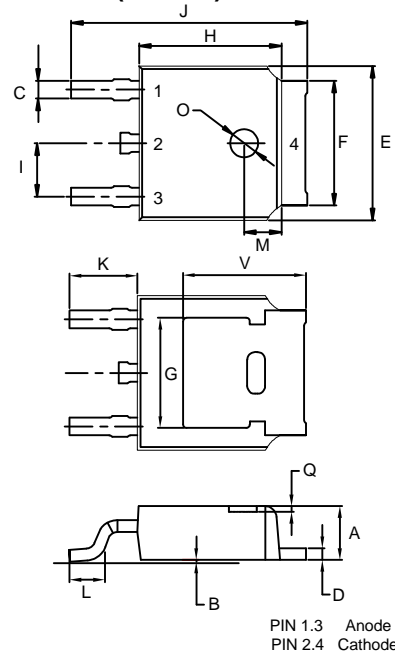
(TO-252) DPAK
