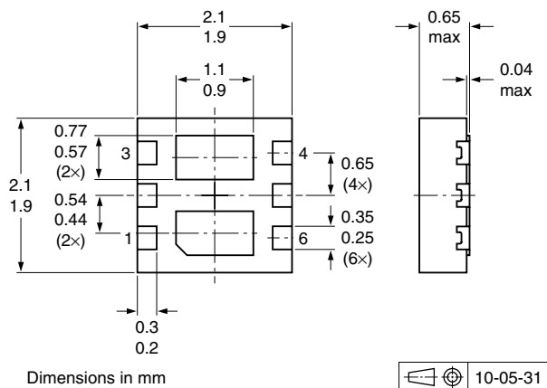
Fig 28. Package outline SOT1118
