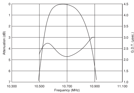
SFELF10M7EA00-B0
