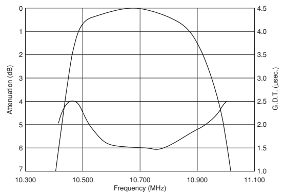
SFELF10M7DF00-B0
